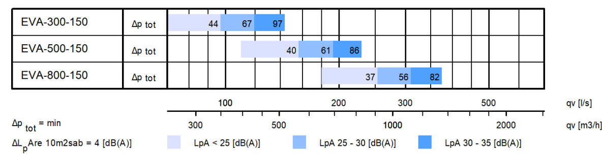
Fig.1. Without plenum
