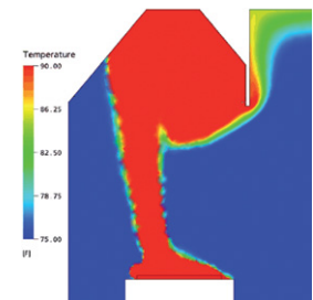
Digitale Simulation der Effizienz der Capture Jet™-Technologie durch die Verbindung von zwei Düsenreihen
