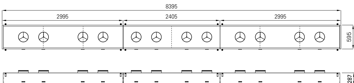
LFU/H - Montage-Beispiel
