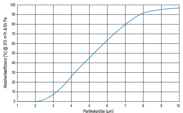
Effizienzcurve der TWIN-FC-Abscheider nach der Methode VDI 2052 (Teil 1) „Raumluftechnische Anlagen für Küchen“. Bestimmung der Rückhalteeffizienz von Aerosolabscheidern in Abluftanlagen von Küchen“
