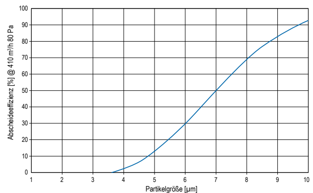
Effizienzcurve der FC Filter nach VDI 2052 (Teil 1) «Raumluftechnische Anlagen für Küchen- Bestimmungen der Rückhalteeffizienz von Aerosolabscheidern in Abluftanlagen von Küchen»
