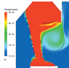
Digitale Simulation der Effizienz der Capture Jet™-Technologie durch die Verbindung von zwei Düsenreihen
